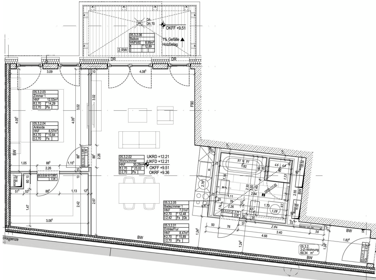
Grundriss 3. Obergeschoss
